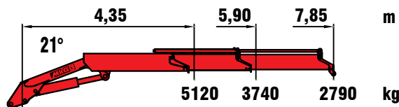
a2 8,05 m max. hydraulische Reichweite (Arm gestreckt) / max. outreach (horizontal position)
